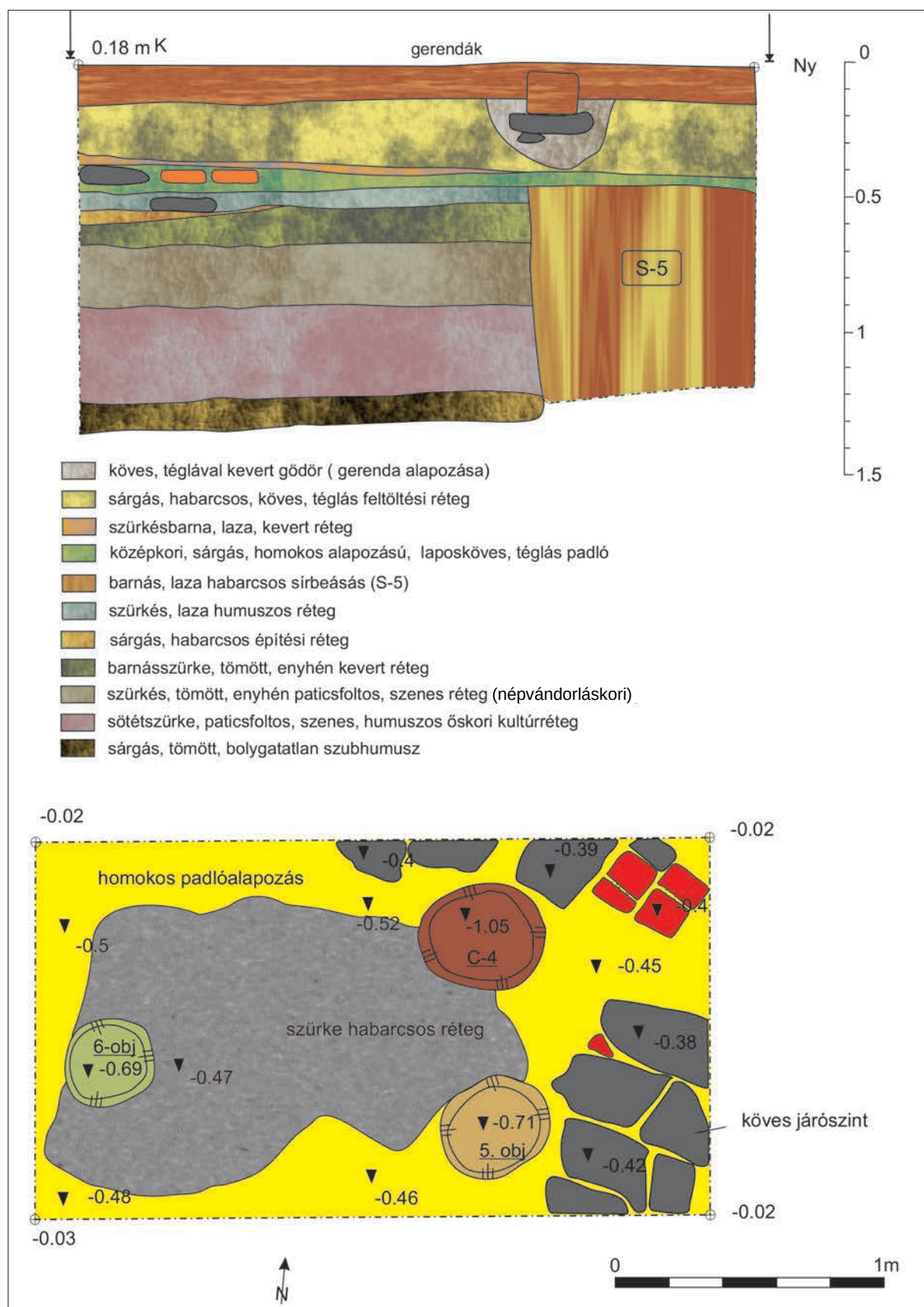
13. ábra A 4. szelvény felszín- és metszetrajzai
