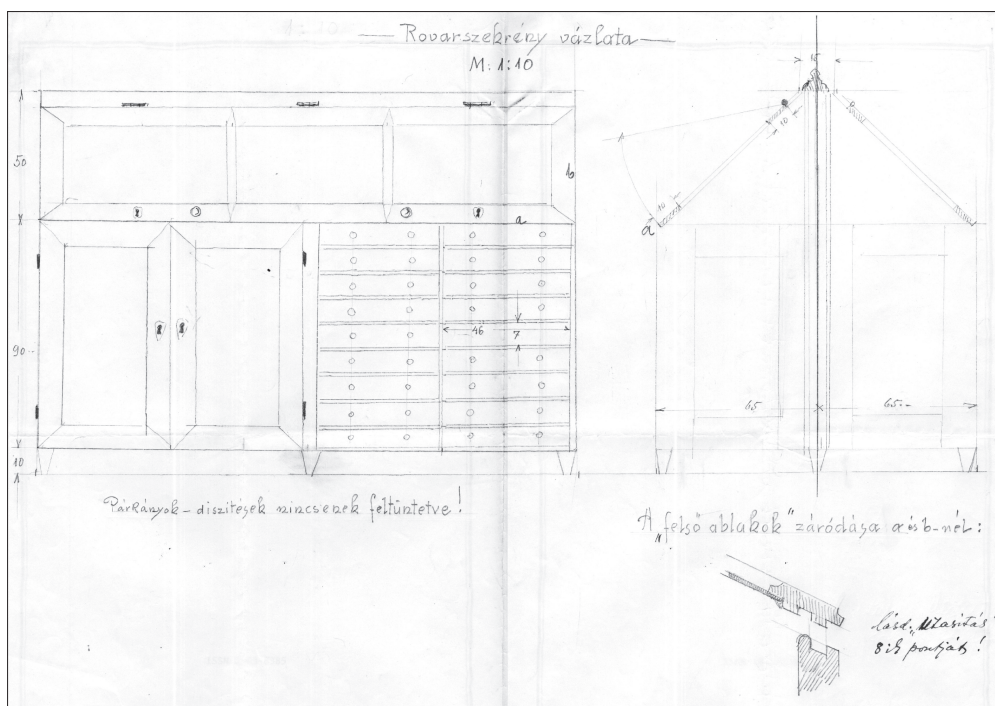
3. ábra A Székely Nemzeti Múzeum rovarszekrényének Köntzei Gerő-féle tervrajza (1936)
